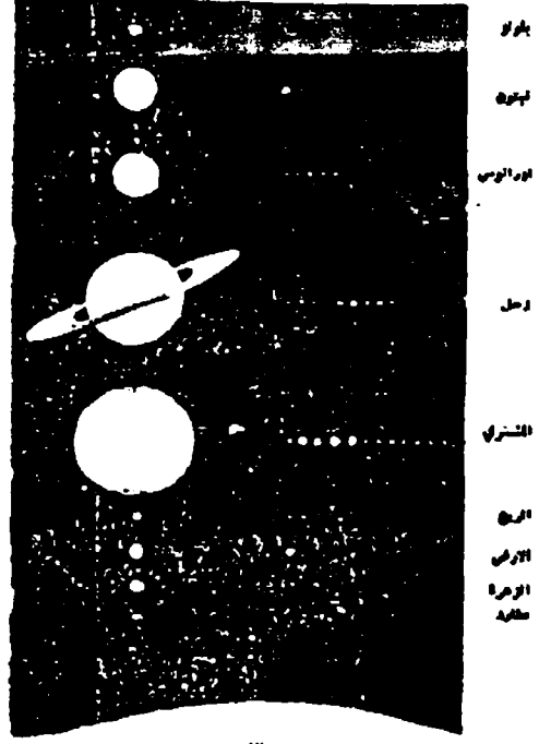
رسم تخطيطي للمجموعة الشمسية
